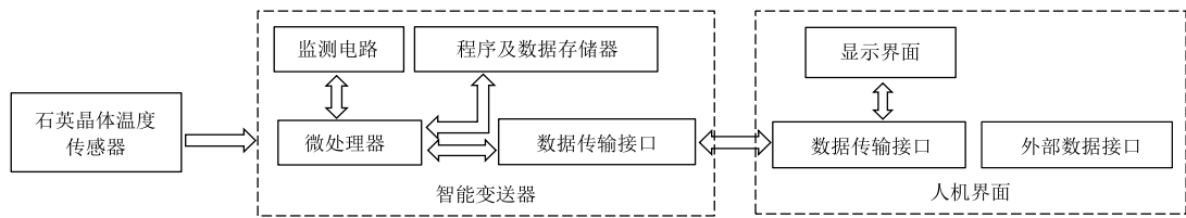
图 1 智能石英温度观测仪结构
